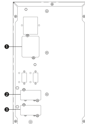
ОСНОВНАЯ СХЕМА. 1. Крышка сменного предохранителя. 2. Входной разъем. 3. Выходной разъем батареи
