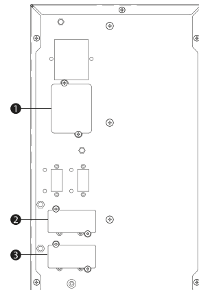
ОСНОВНАЯ СХЕМА. 1. Крышка сменного предохранителя. 2. Входной разъем. 3. Выходной разъем батареи
